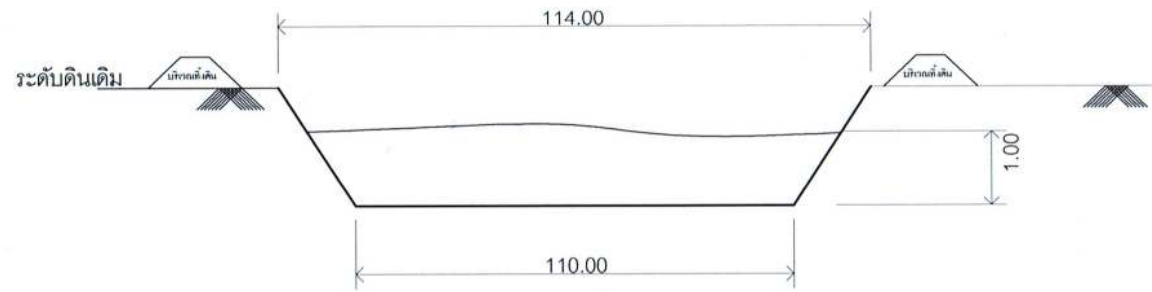
รูปตัดยาวทั่วไป SCALE 1:100
