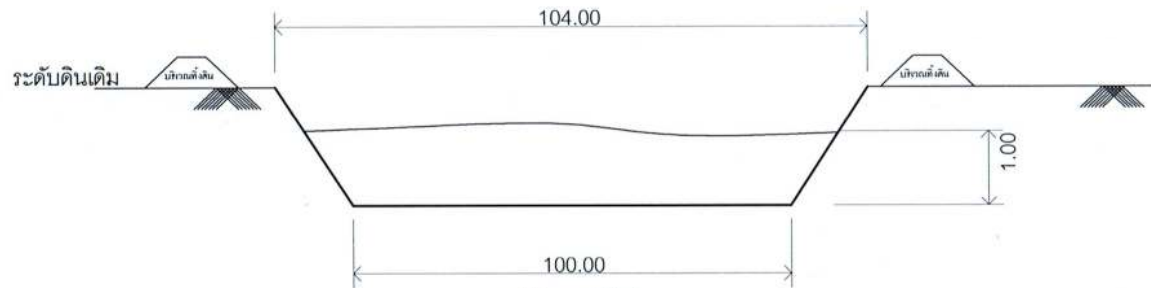
รูปตัดขวางทั่วไป SCALE 1:100
