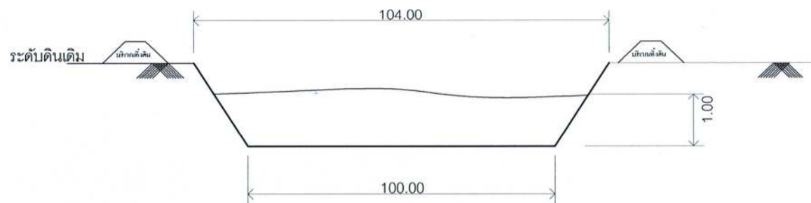
รูปตัดยาวทั่วไป SCALE 1:100
