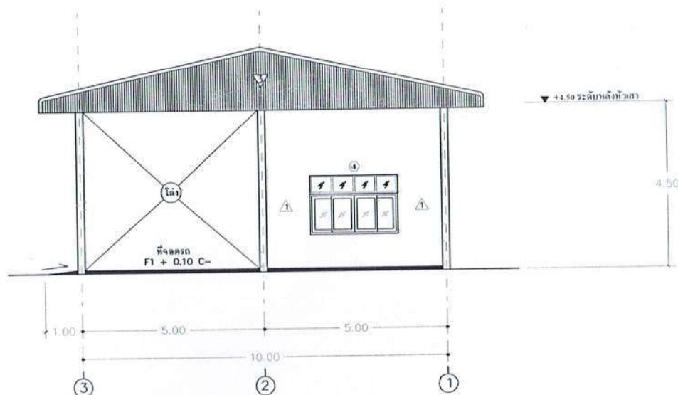
รูปด้าน ④ SCALE 1: 100
