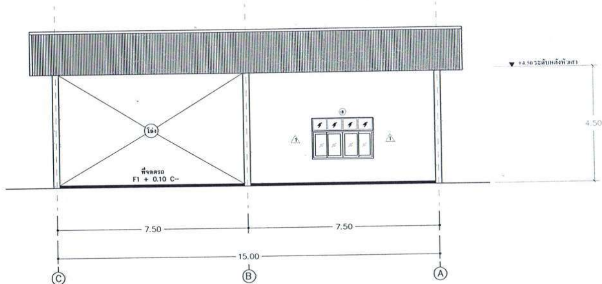
รูปด้าน ③ SCALE 1: 100
