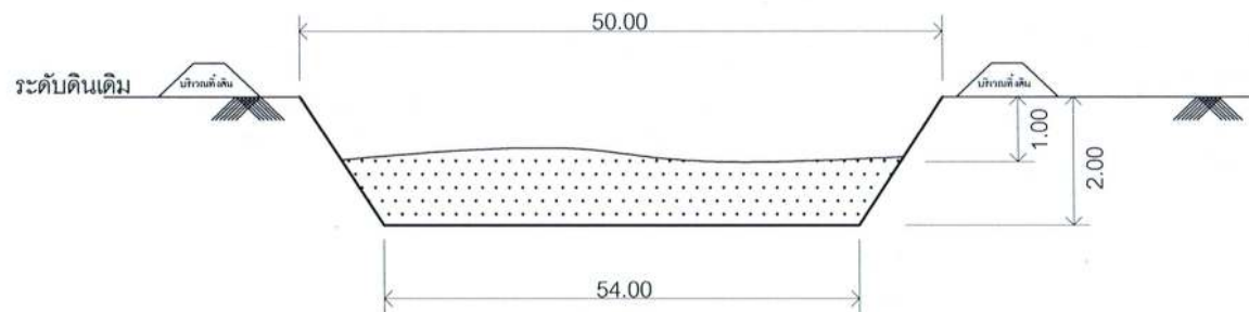
รูปตัดขวางทั่วไป SCALE 1:500
