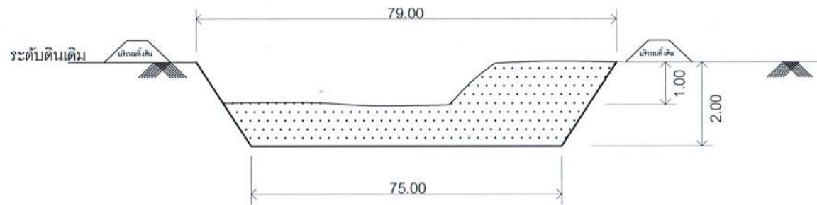
รูปตัดยาวทั่วไป SCALE 1:500
